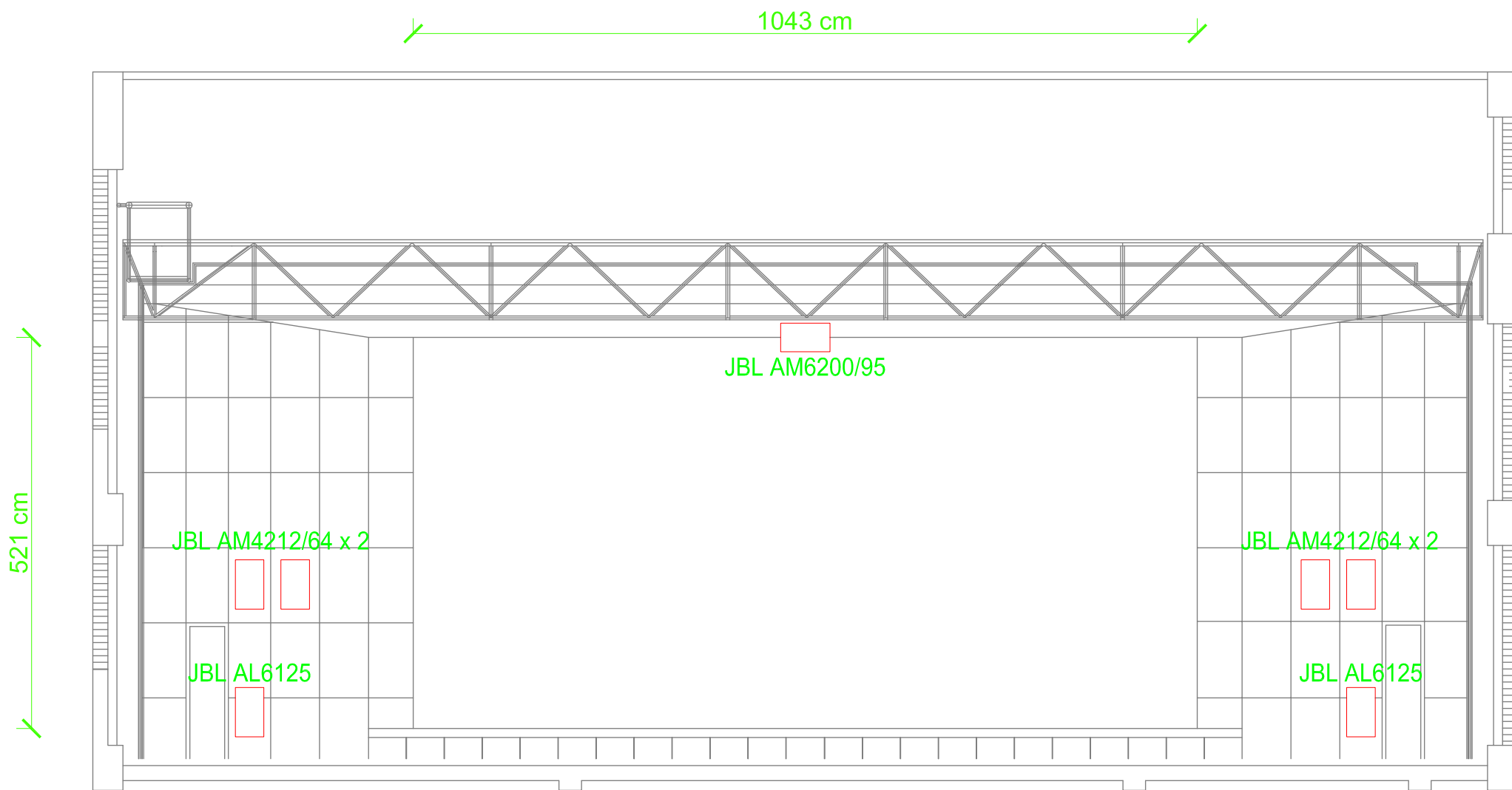
ZVUČNIČKI SUSTAV - PRESJEK SOUND SYSTEM - CROSS SECTION
